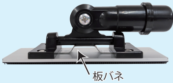
板バネ
